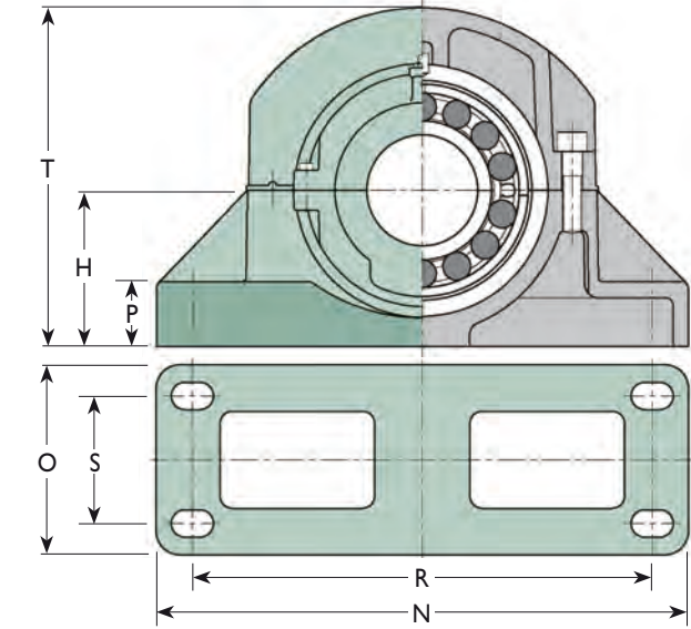
4 Bolt
