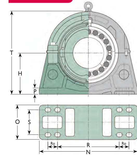
8 Bolt
