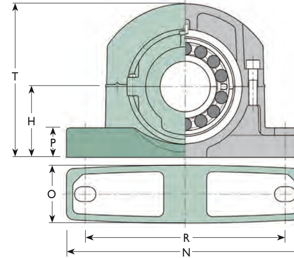
2 Bolt
