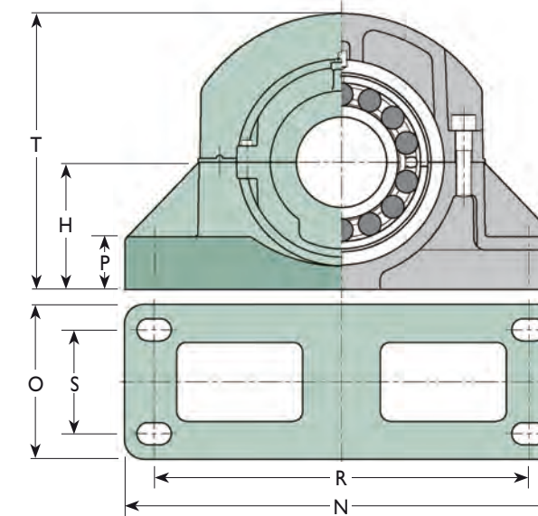
4 Bolt
