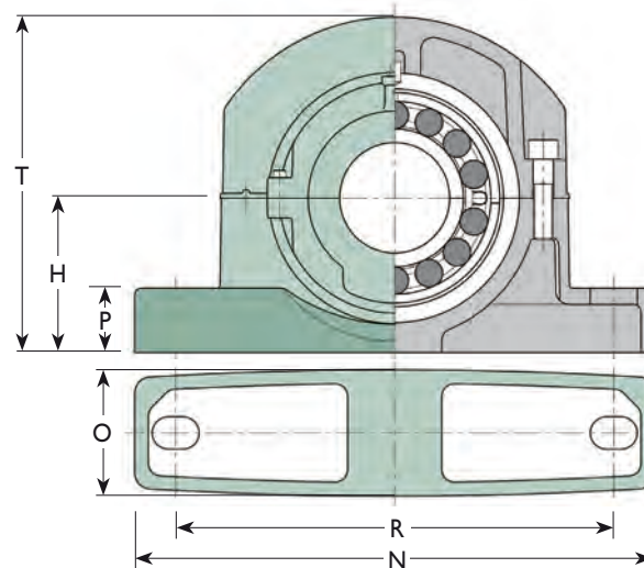
2 Bolt
