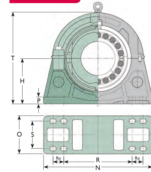
8 Bolt
