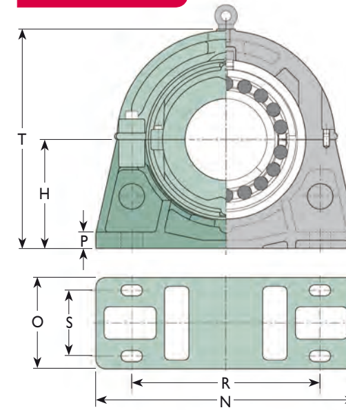
4 Bolt
