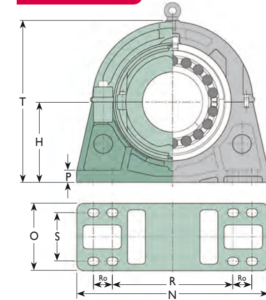
8 Bolt
