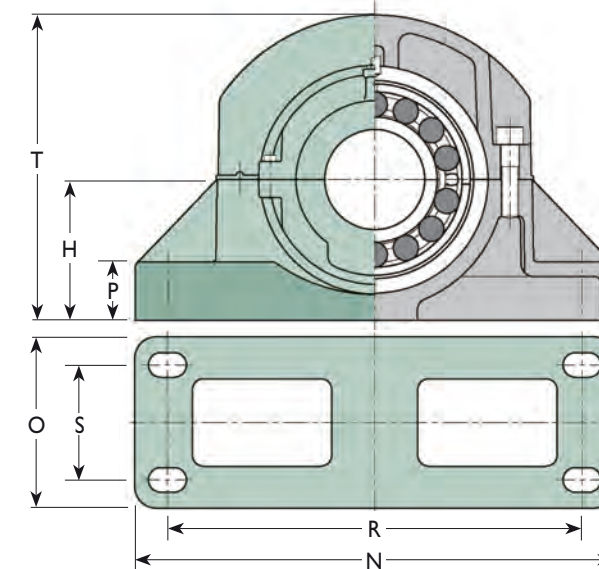
4 Bolt
